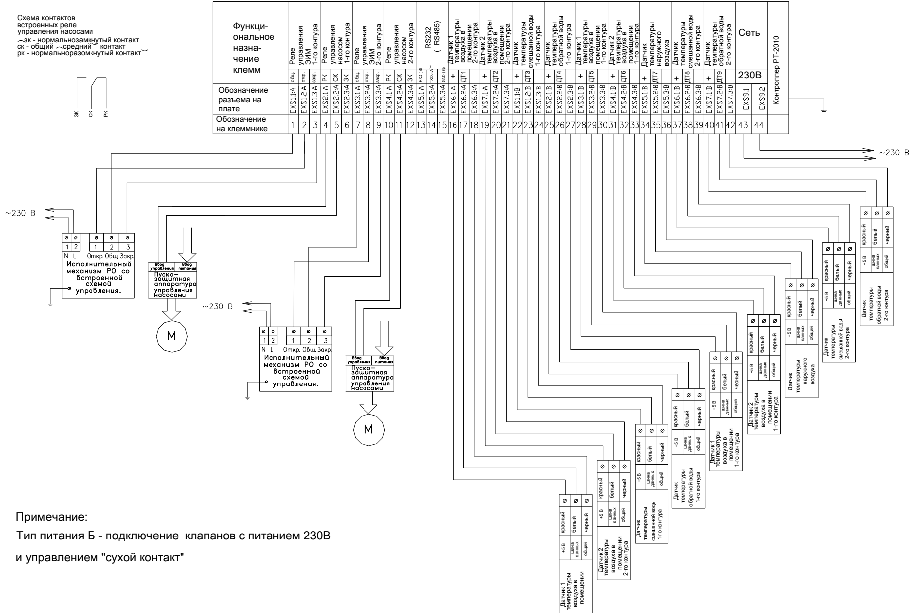
Рисунок 1 Регулятор РТ-2010 тип питания регулирующих органов - Б
