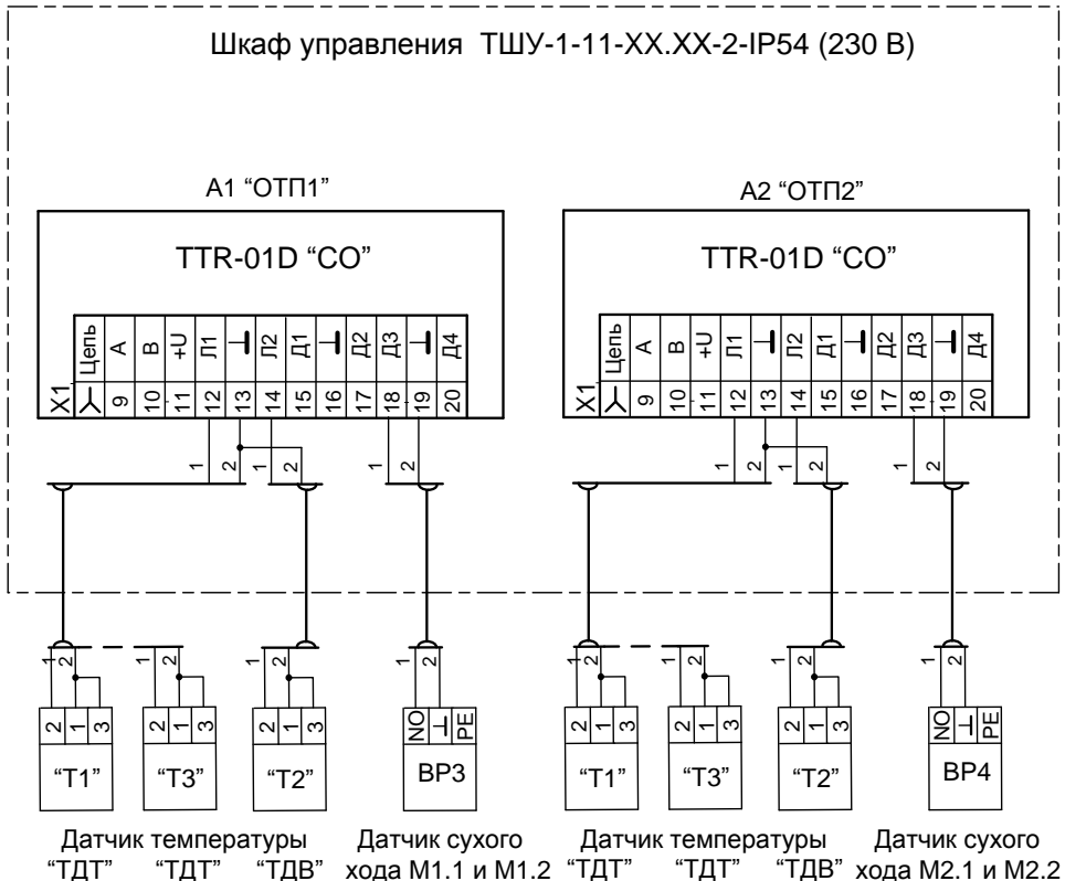
Рисунок Б.3 Схема подключения внешних датчиков
