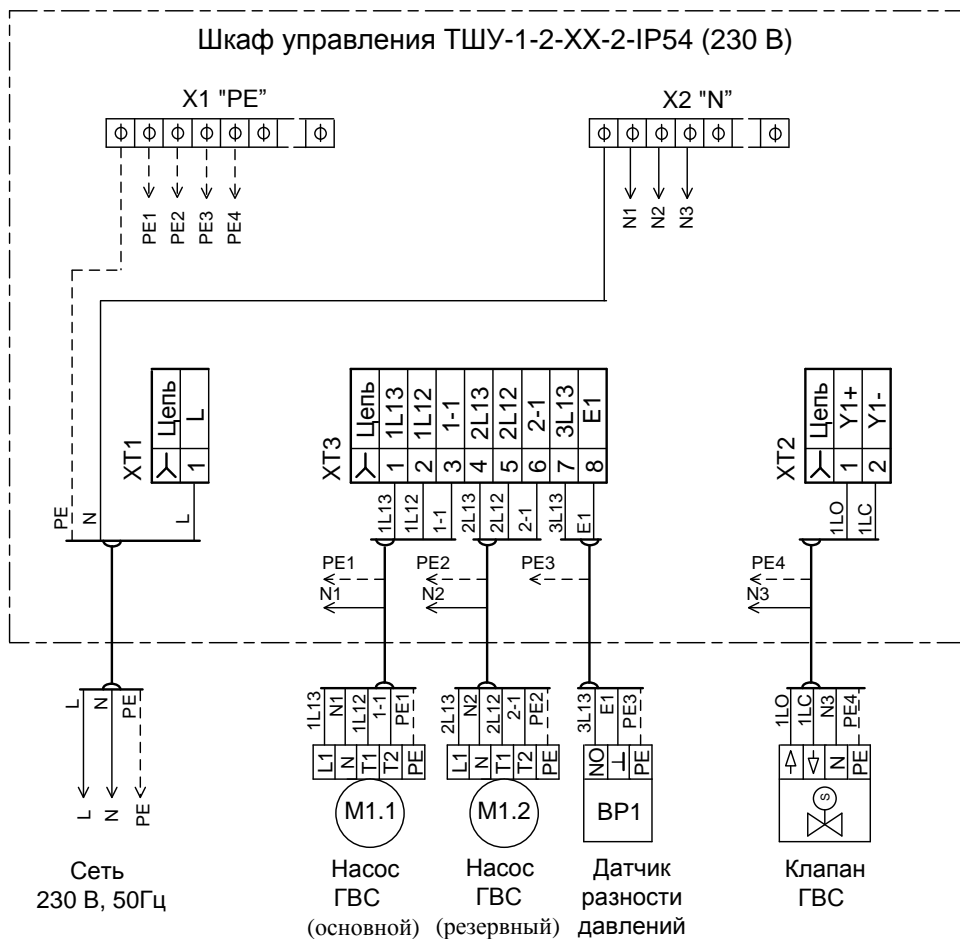
Рисунок Б.1 Схема подключения насосов и клапанов регулирующих
