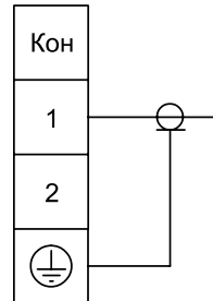
Рисунок 14 Схема подключения кабеля РК-50 к пьезодатчику ПЭП 3-4
