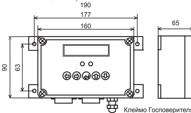
Рисунок 1а - Габаритные размеры УПР и электронного блока
