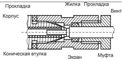
Рисунок 13 - Схема подключения кабеля РК-50 к пьезодатчикам ПЭП 3-1 и ПЭП-6-1
