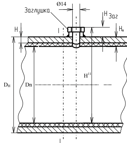
Рисунок 4а Эскиз к методике измерения суммарной толщины стенки трубопровода и отложений.
