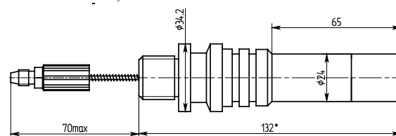
е) ПЭП типа ПЭП-3-65
