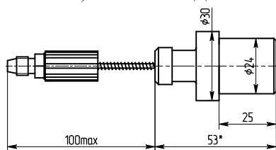
в) ПЭП типа ПЭП-3-25
