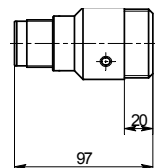
а) Бобышка УСД
