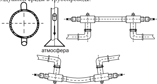
Рисунок 2 Примеры неправильного расположения измерительного участка
