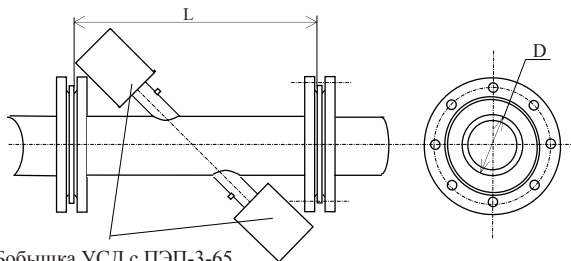
Бобышка УСД с ПЭП-3-65
