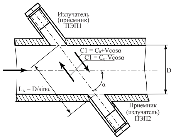
Рисунок 4 - Принцип работы теплосчетчика
