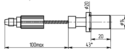
ж) ПЭП типа ПЭП-6-20
