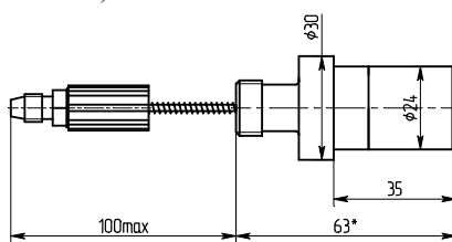
г) ПЭП типа ПЭП-3-35
