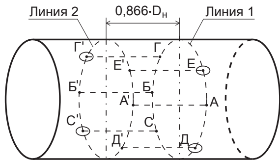
Рисунок 8 - Разметка трубопровода при врезке по хорде,
