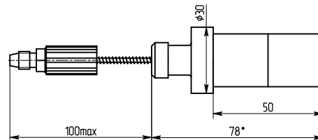
д) ПЭП типа ПЭП-3-50
