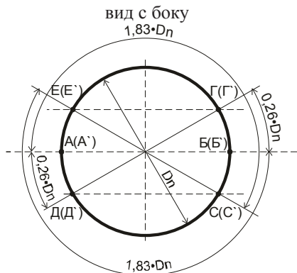
Рисунок 9 - Разметка УПР при врезке по хорде вид с торца
