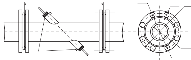
ПЭП-6-20; ПЭП-3-25; ПЭП-3-35; ПЭП-3-50.
