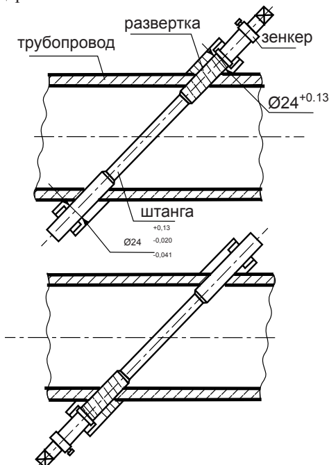
Рисунок 6 - Схема доработки отверстий
